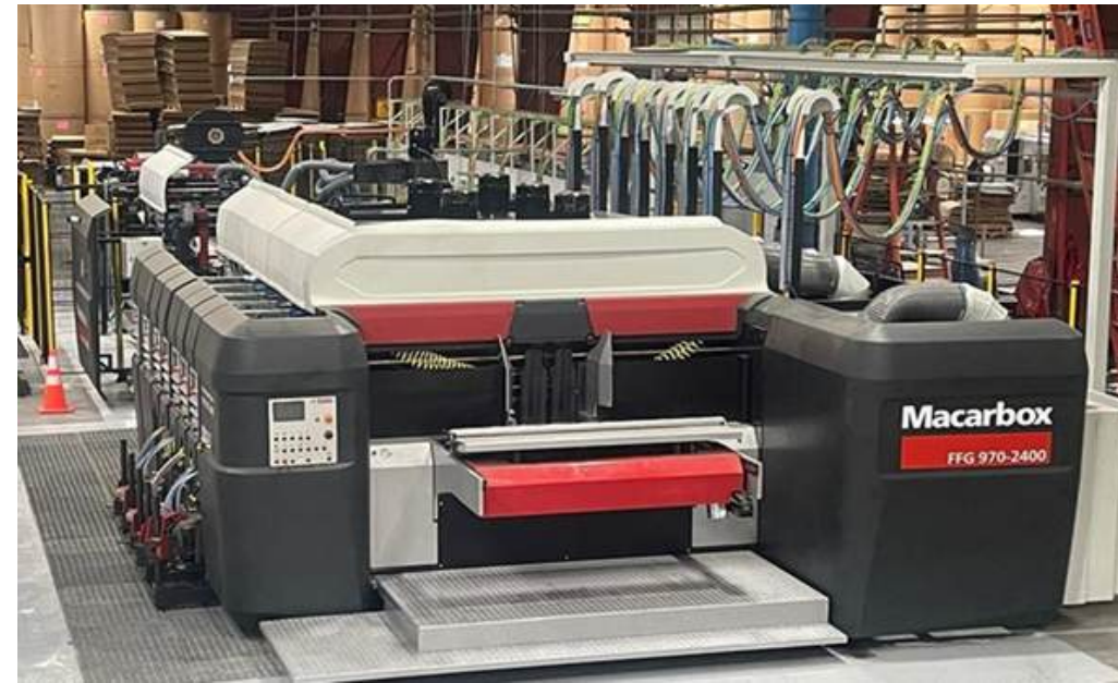
CANASA: Máquina FFG Macarbox 970 / 2400 Puesta en marcha: Septiembre 2024
